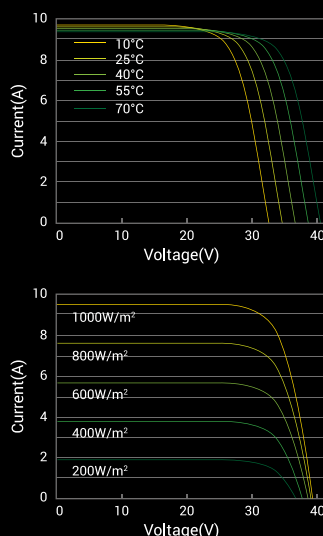
I-V Curve: (A-P340)
